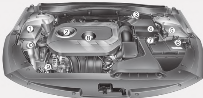
■ موتور بنزینی (۲ لیتری - MPI)
